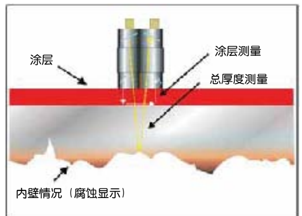
Krautkramer的TopCOAT技术: TopCOAT探头(具有两个接收晶片和两个发射晶片), 能够一次测量即确定涂层厚度和母材厚度, 而不需要多次回波测量厚度。
