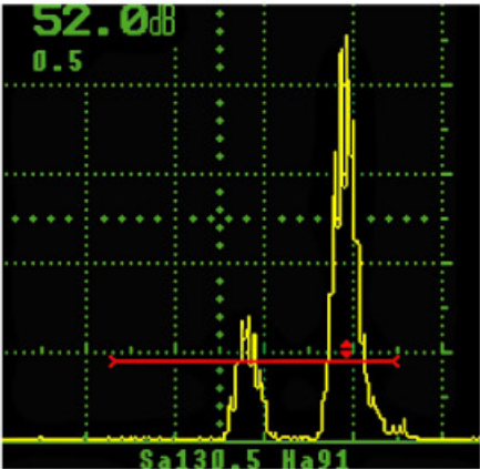
峰值：测量闸门内最高回波的声程和波幅。
