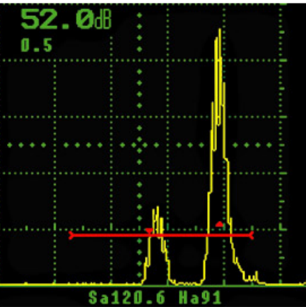
波前：测量闸门内第一个回波的声程，测量闸门内最高回波波幅。
