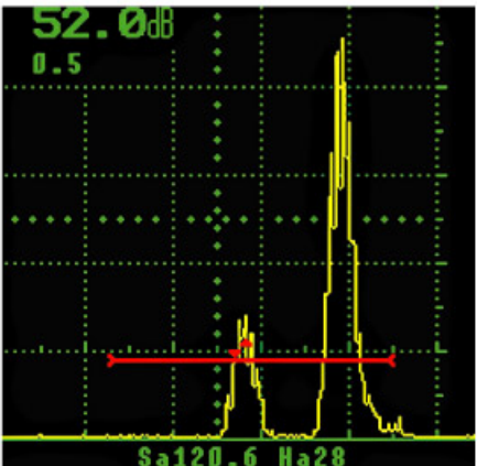
JFlank：测量闸门第一个回波的声程和波幅。
